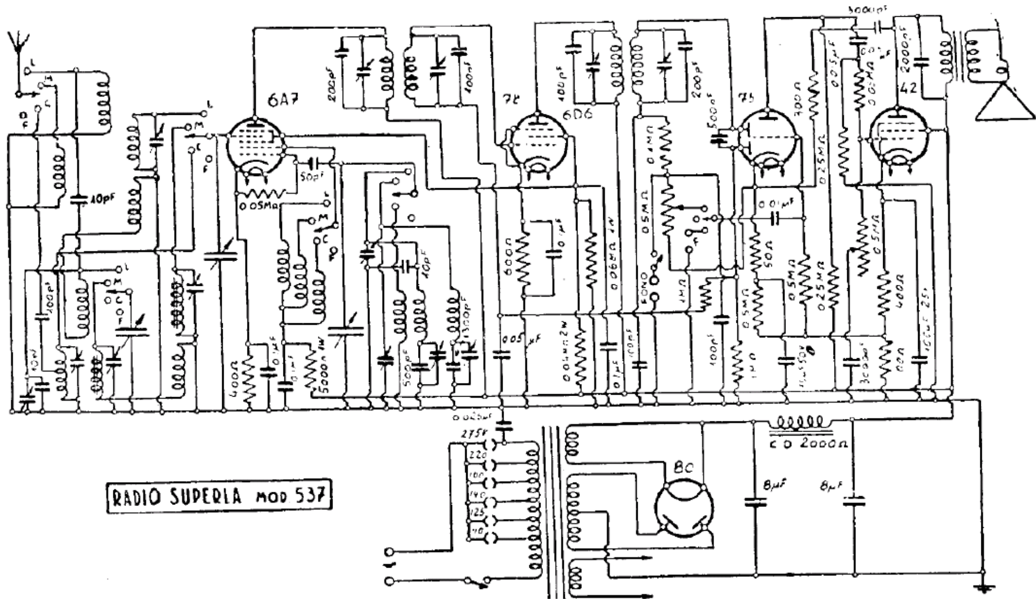
RADIO SUPERLA — Modelli « 537 » e « 1537 » - Produzione 1938. Media frequenza: 128,25 kHz.
